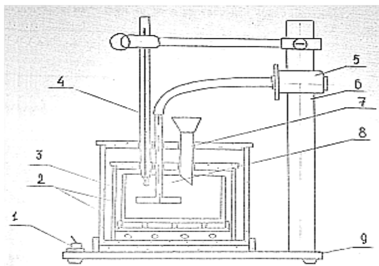
Рис. 1. Схема калориметра:
